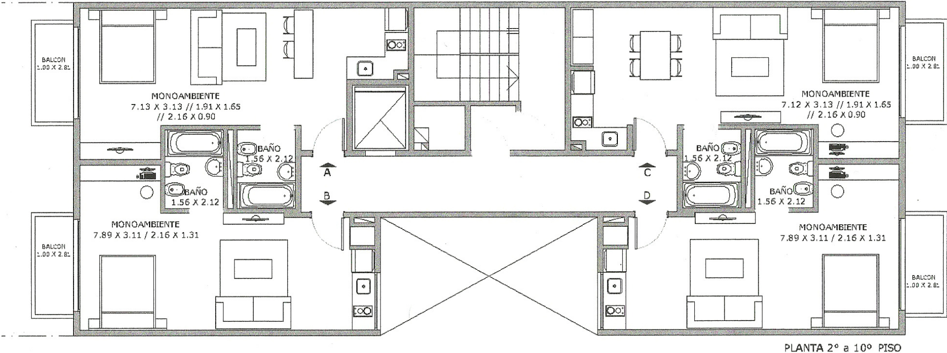
PLANTA 2º a 10º PISO
